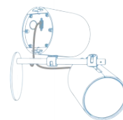
Konsole mit 2x AS-3/5
